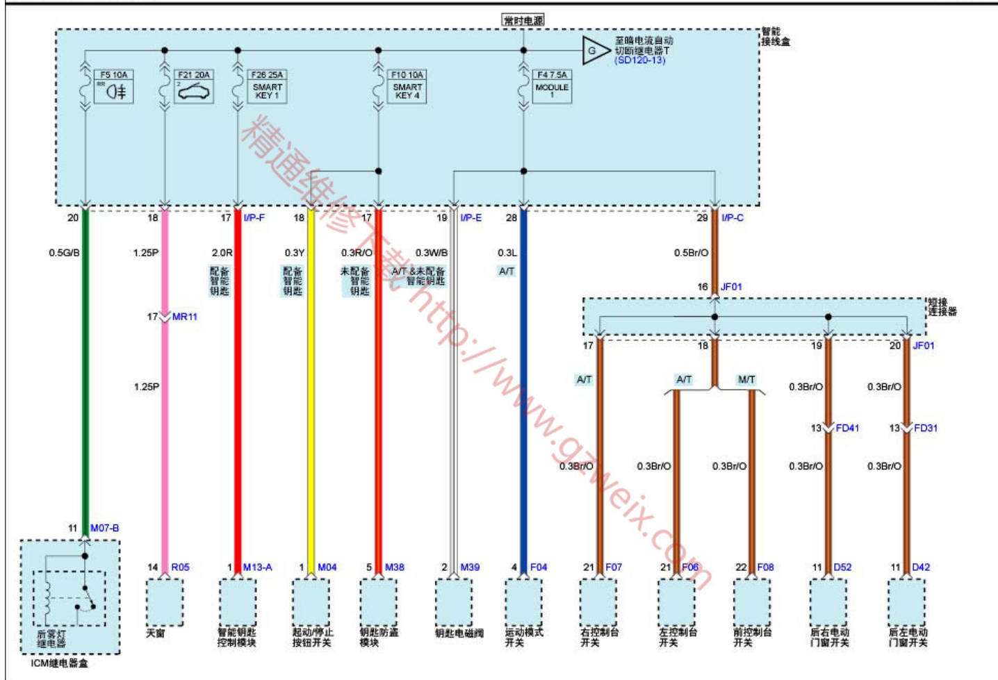
室内保险丝分布(12)
